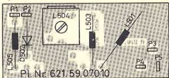
Bestückungsseite
