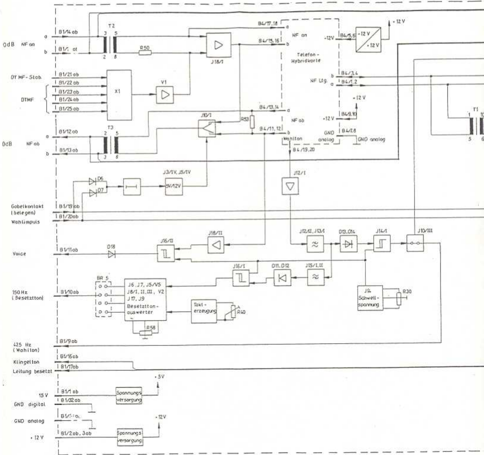
Blockschaltbild:
