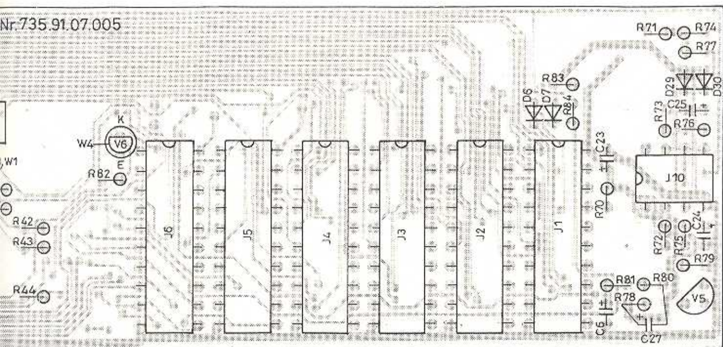
Bestückungsseite
